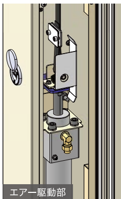
エア駆動部
