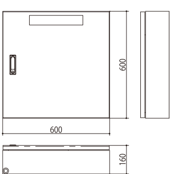
防爆仕様コントローラー 【外観寸法図（電気コントローラー）】
